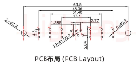
PCB布局 (PCB Layout)
