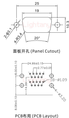
PCB布局 (PCB Layout)
